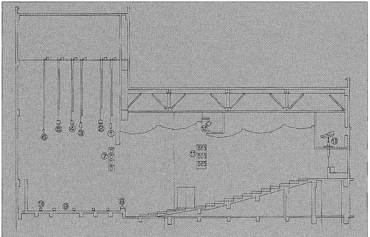
ホール断面図
