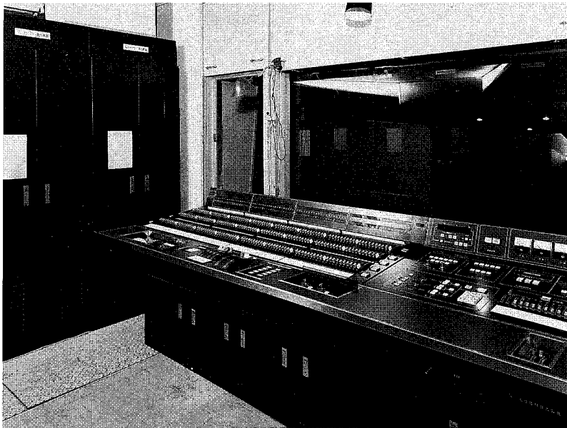
大ホール調光卓とサイリスター調光器盤
