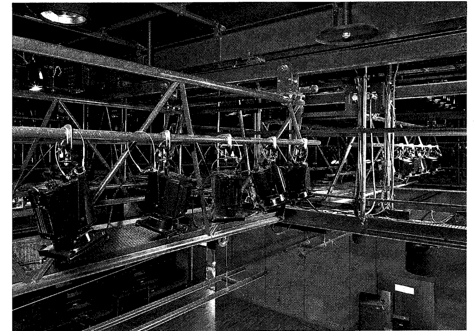
走行ブリッジと昇降ボタンによって、スポットライトの位置は自由に設定できます。
