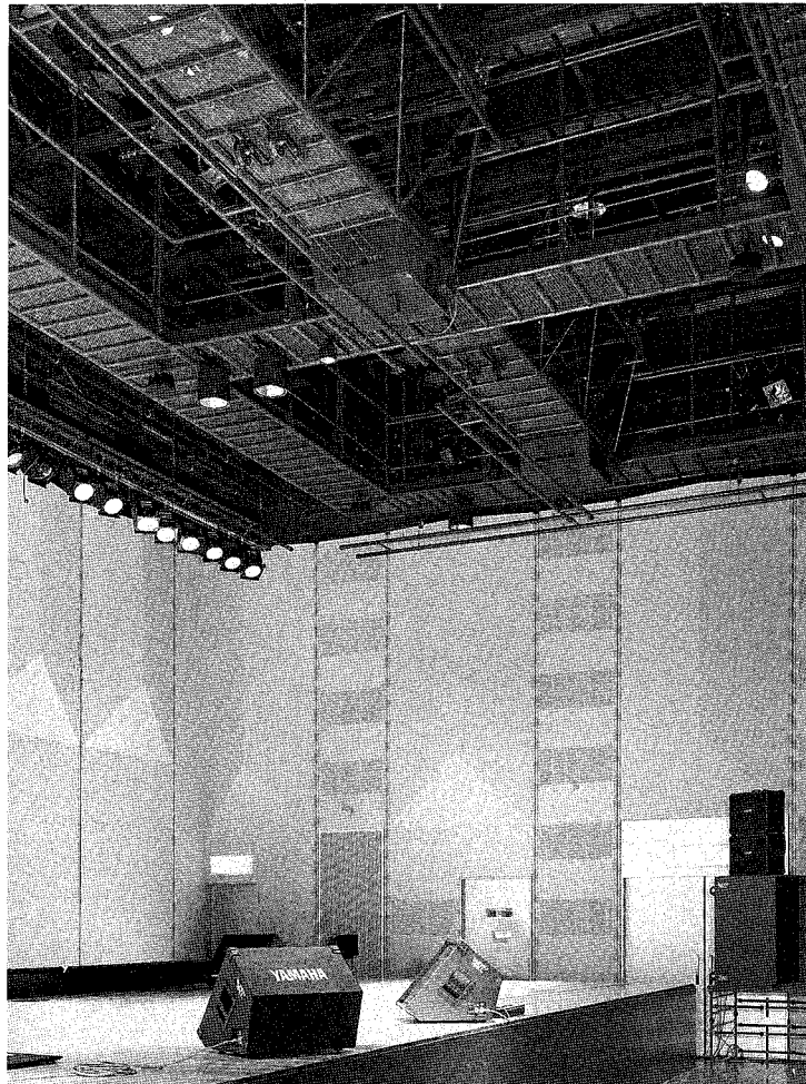
どの位置に舞台が設定されても、同じ条件でライティングができるように、ホールの上全面には固定ブリッジと12本の走行ブリッジが設置されています。
