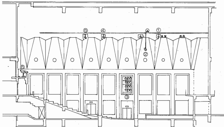
主ホール断面図
