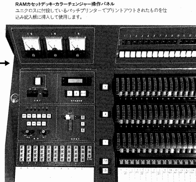
RAMカセットデッキ・カラーチェンジャー操作パネル
