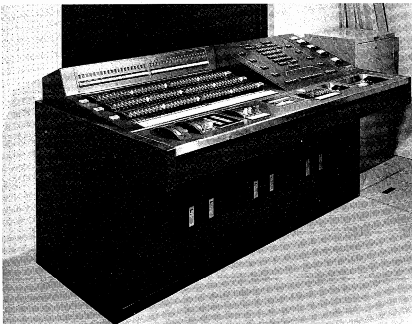
調光室の照明操作卓と電子クロスバー選択操作卓
