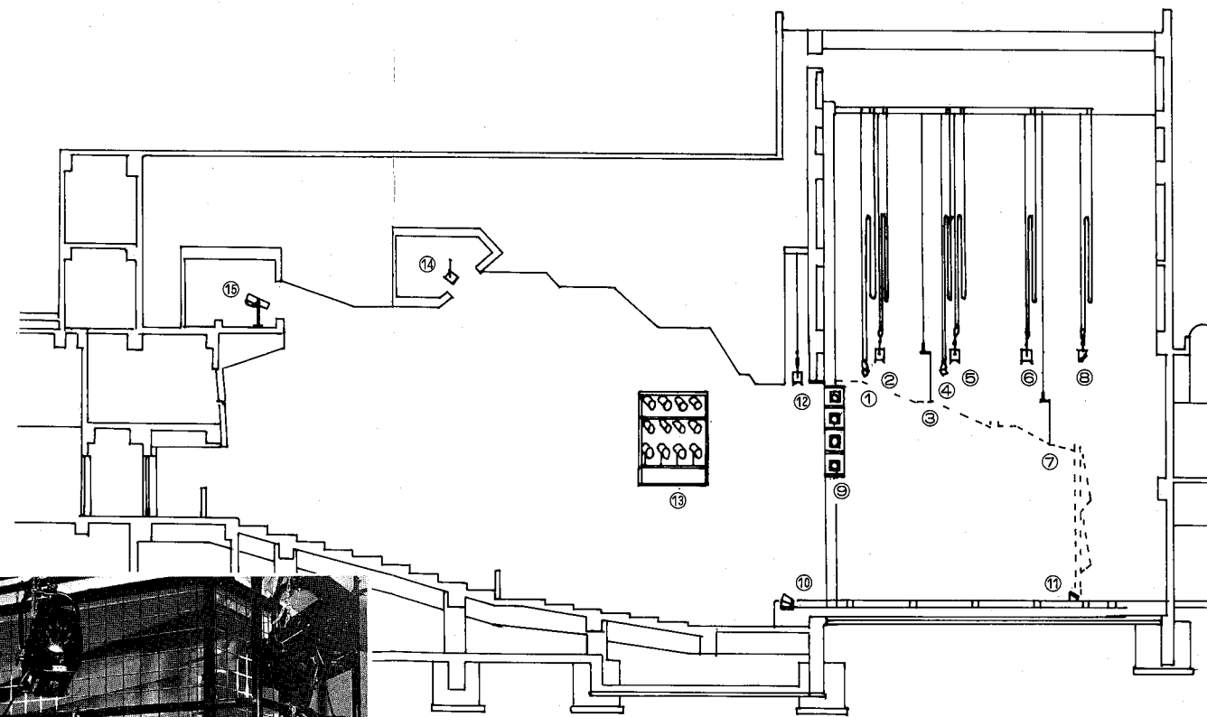
ホール断面図
