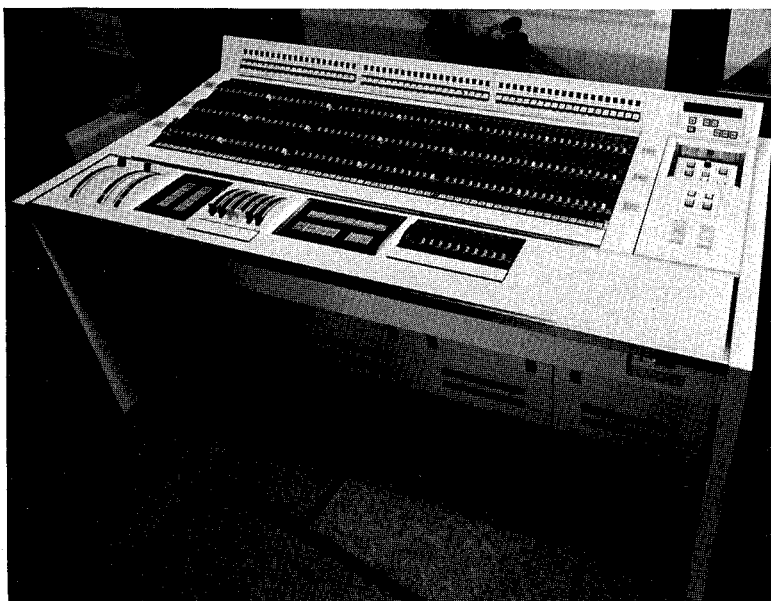
調光室の照明操作卓
