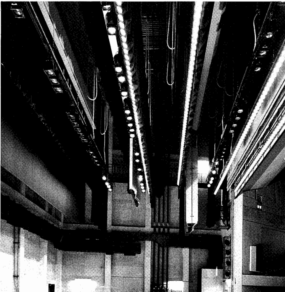
舞台上部
