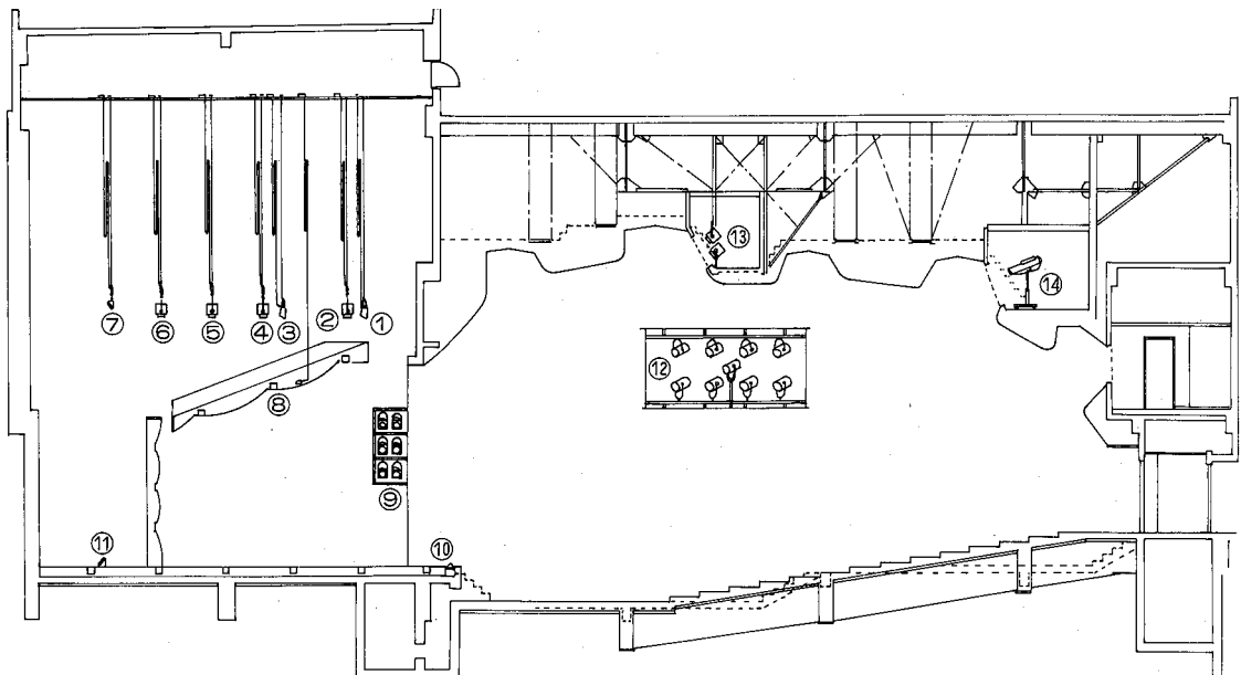
ホール断面図
