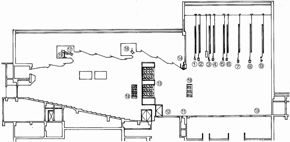
大ホール断面図
