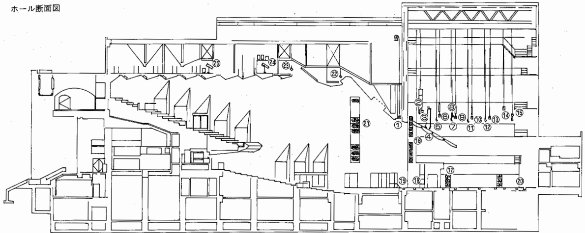
ホール断面図
