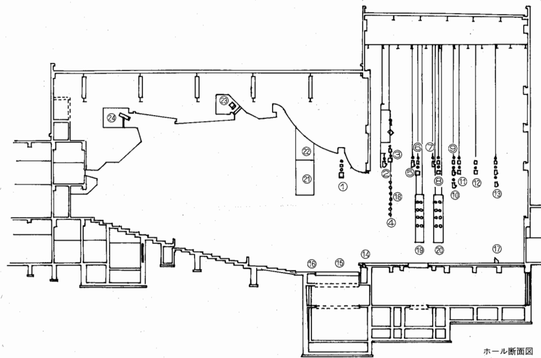
ホール断面図
