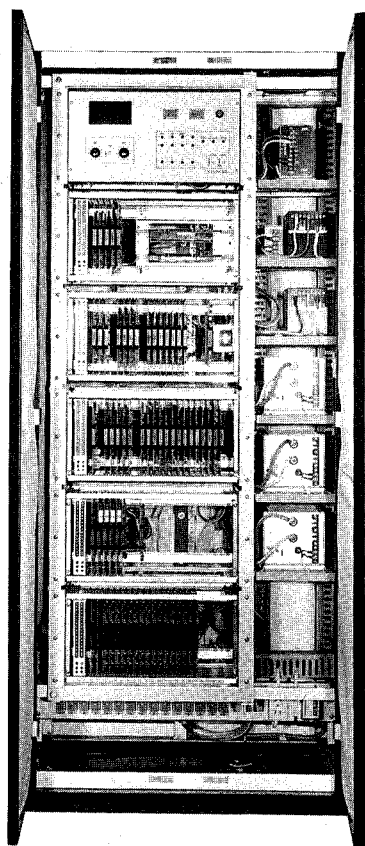
記憶処理盤
