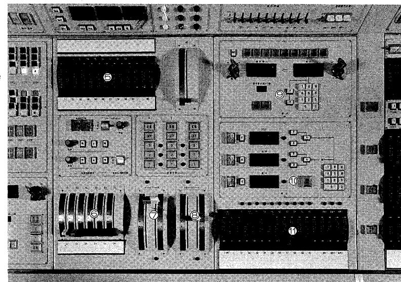
⑤シーケンスディーマー用フェーダー ⑥グループフェーダー (G1~G6) ⑦クロスフェーダー (CF A-B) ⑧クロスフェーダー (CF AB-C) ⑨書込みパネル ⑩読出しパネル ⑪フリーフェーダー (F-MF×1/PF×10)
