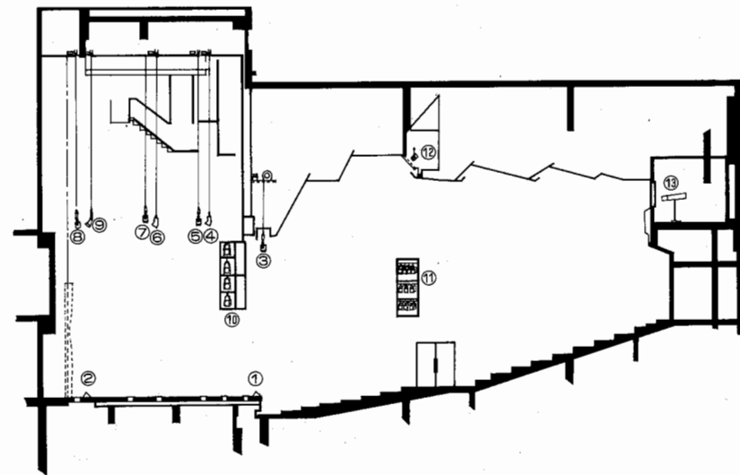
ホール断面図
