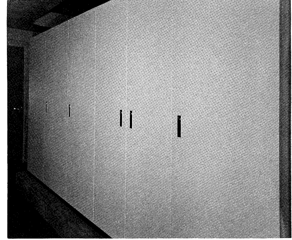
■サイリスター調光器盤(大ホール) 1基 舞台用6kWサイリスター 34台 客席用6kWサイリスター 6台
