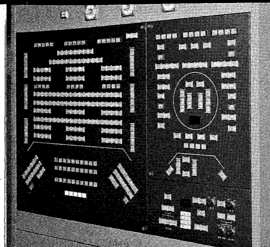
電子クロスバー選択操作盤
