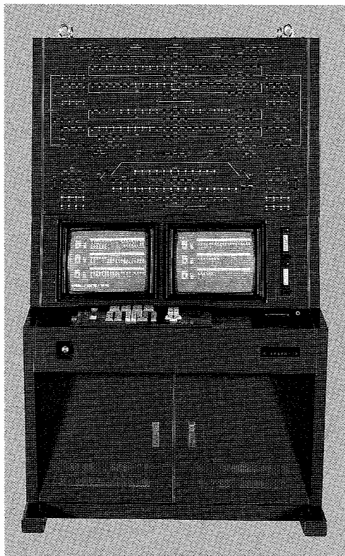
回路選択操作盤(ユニクロスCRT表示式)
