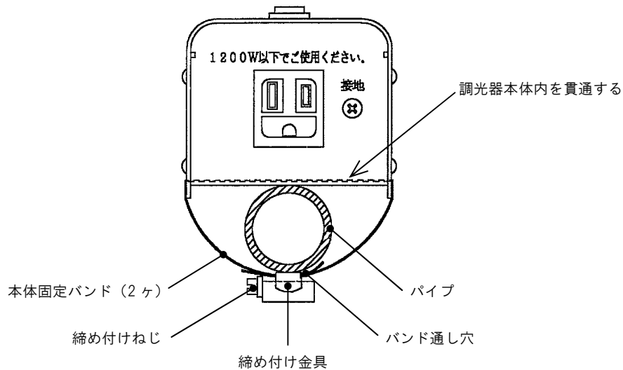
パイプアームへの取付例
