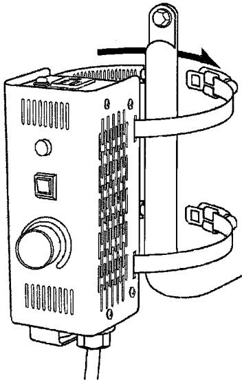
パイプアームへの取付例
